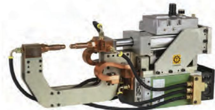
Сварочные клещи для роботови ручной сварки с возможностью перемещени
